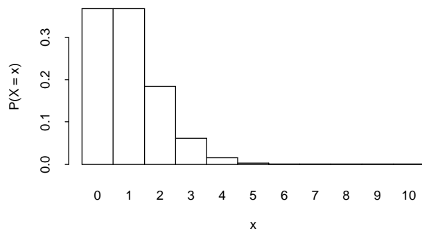
Poisson Prob. Fun., mu=1
