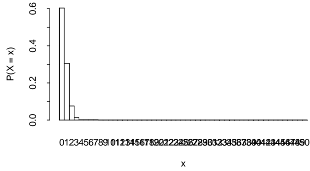
Binomial Prob. Fun., n=100, p=.01
